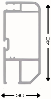
Bug Screen 66mm AST26- WH
