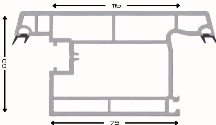
Casement Door Sash AST06-WHG
